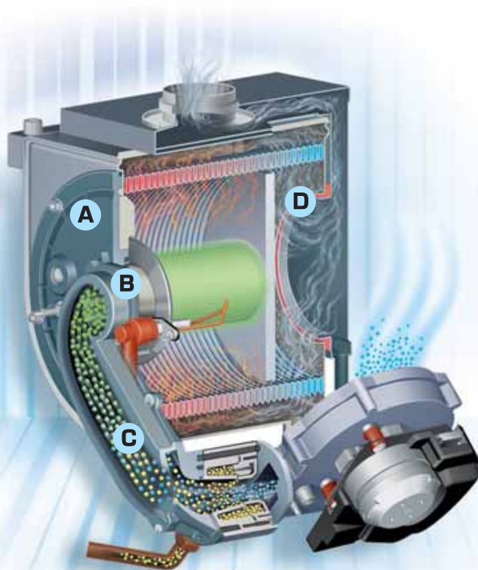
Il sistema premiscelato a condensazione Murelle HE ad accumulo
